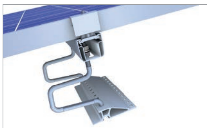
Dubbele dakhaak voor hoge sneeuwbelasting
